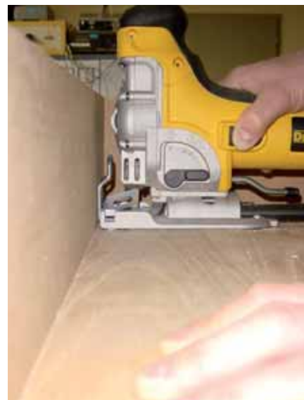
Randnahe Schneiden bis zum Anschlag des Sägeschuhs mit dem HCS-Sägeblatt DT2074.
